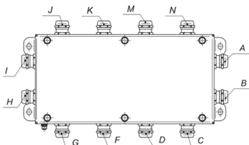
KM-O IP66 1530, KM-O IP66 1530 «Север», FEJBG1530 IP66
